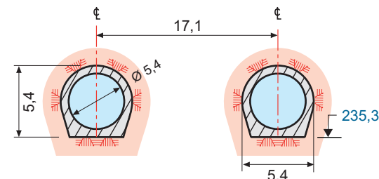
Conduites forcées – Coupe C
