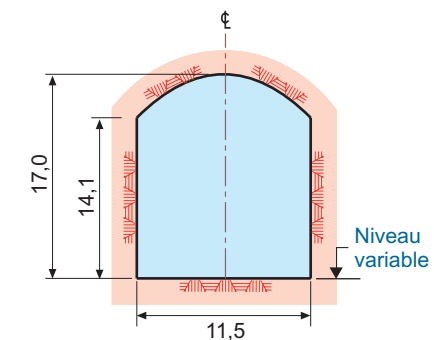
Galerie d'aménée – Coupe B
