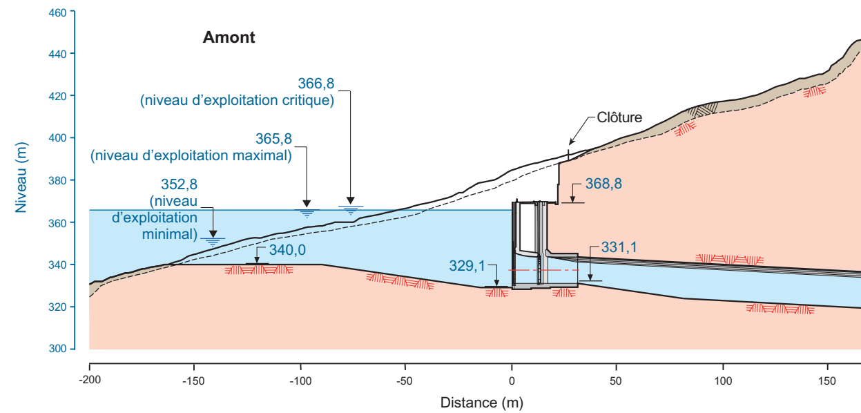
Prise d'eau – Détail 1
