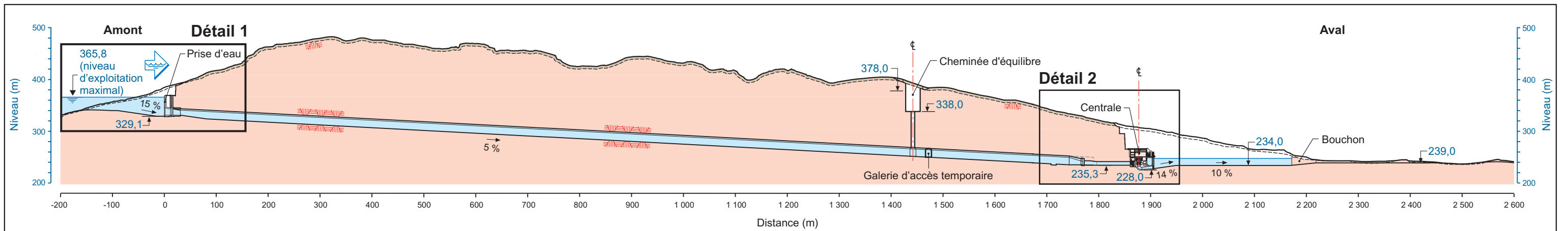
Ouvrages de production – Profil longitudinal A
